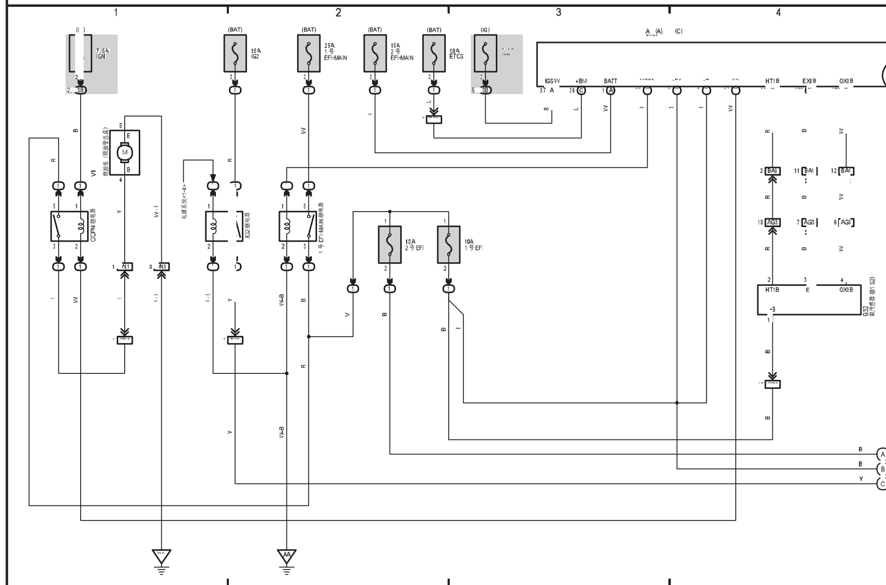
发动机控制系统 (6ZR-FE)
